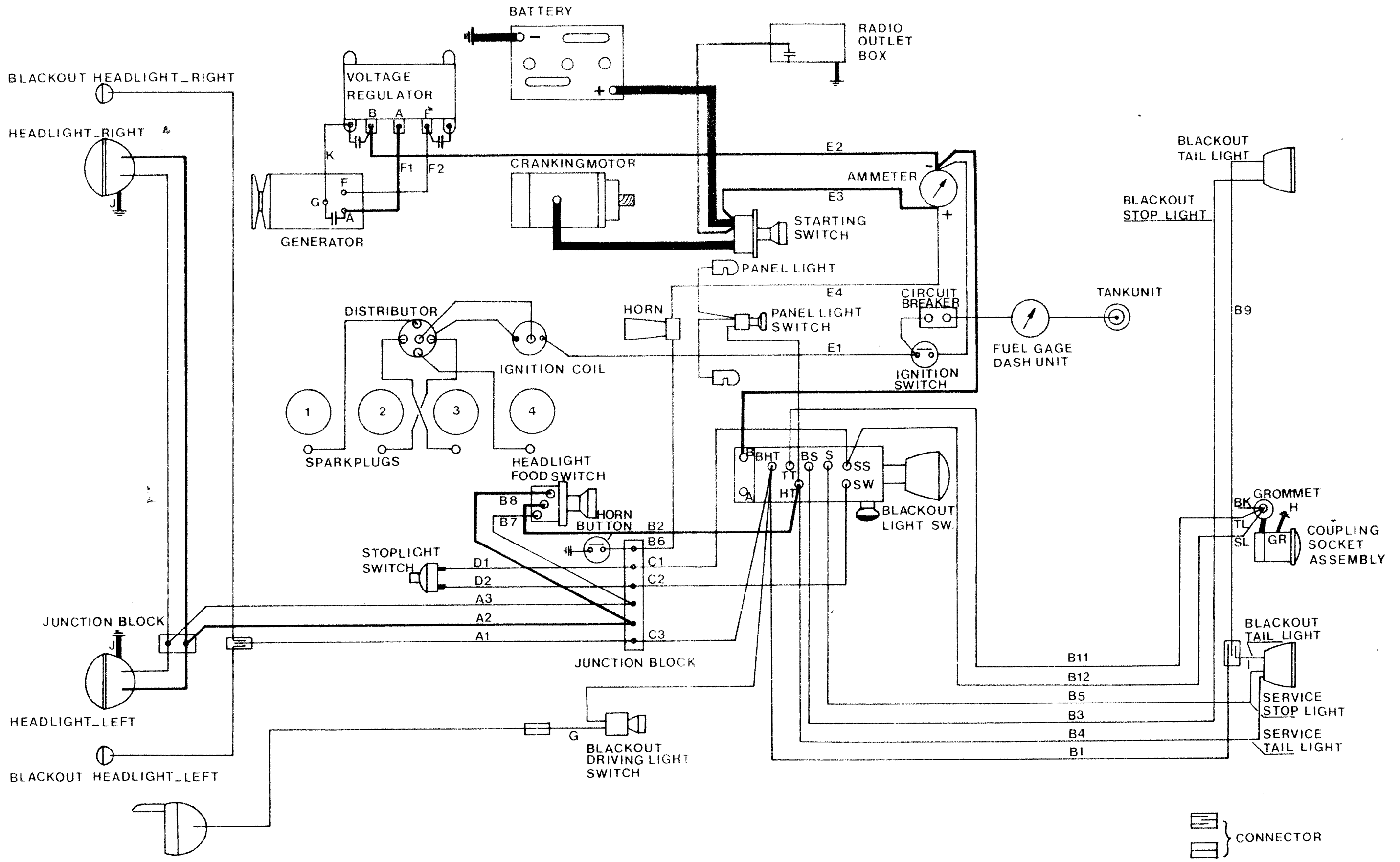
JEEP_WIRINGDIAGRAM
